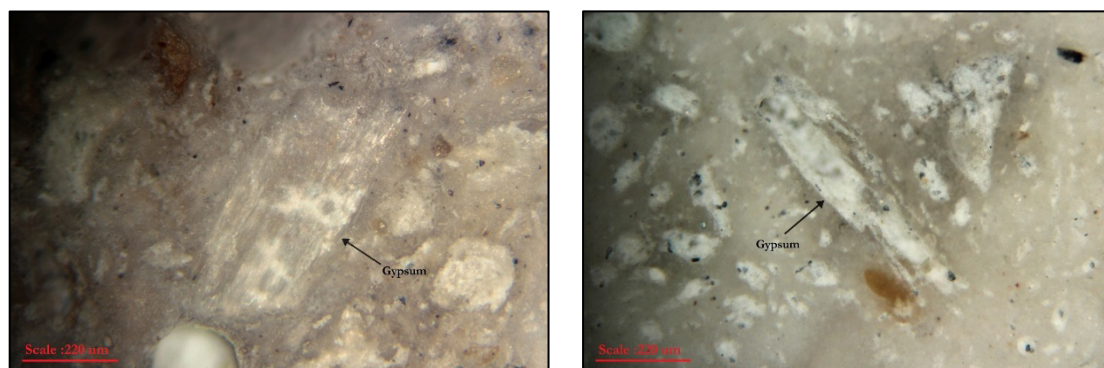
شکل ۷. بلورهای کشیده و درشت‌دانه ژیس در ماتریس کربناتی نمونه‌های MLA.K.1 (چپ)، ZAR.A.1 (راست)
