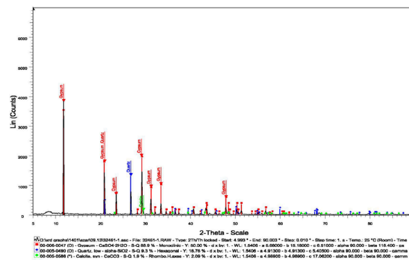
شکل ۲. الگوی XRD نمونه A Figure 2. XRD pattern of sample A
