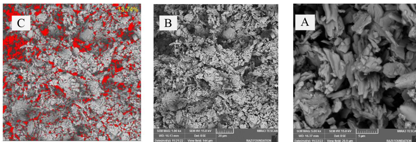
شکل ۸. میکروگراف‌های SEM مربوط به نمونه A در دو بزرگنمایی (A) ۱۰۰۰، (B) ۵۰۰۰ برابر و (C) تصویر پردازش شده جهت اندازه‌گیری درصد تخلخل
