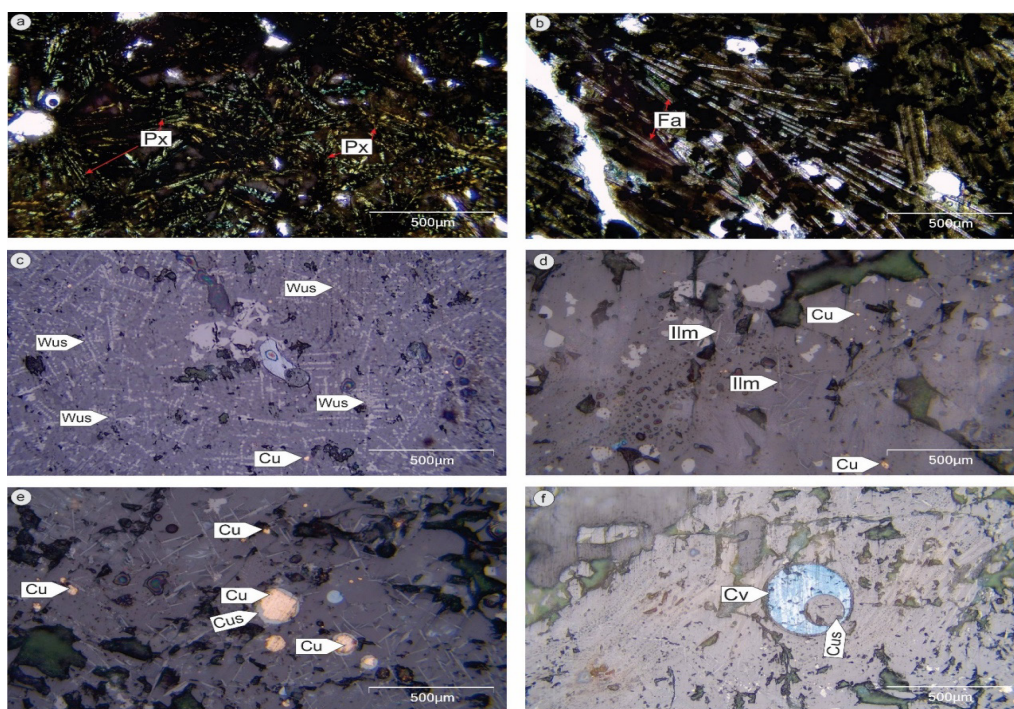
شکل ۶. (a) کانی پیروکسن به صورت بلورهای دم‌چلچله‌ای و به رنگ سبز (b) کانی الیوین به صورت تیغه‌های کشیده و بی‌رنگ (c) کانی وستیت به صورت بلورهای کشیده و پراکنده در ماتریس (d) کانی ایلمنیت به صورت تیغه‌های بسیار نازک (e) کانی مس نیتئو با حاشیه‌ای از سولفید مس (f) کانی‌های مس به صورت کوولیت و دیگر سولفیدهای مس.
