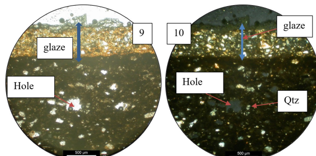
شکل ۹. فتومیکروگراف، نمونه ۹، نور PPL، طول میدان دید 2.7mm، بافت ناهمگن، لایه لعاب در بالای تصویر که دو لایه لعاب شیشه ای همراه با لایه متشکل از کوارتز و مذاب سیلیسی که بر روی بدنه قرار دارد. در این نور فضای خالی به رنگ روشن است. فتومیکروگراف، نمونه ۱۰، نور XPL، طول میدان دید 2.7mm، بافت ناهمگن. همان تصویر ۹ در نور متقاطع است.
