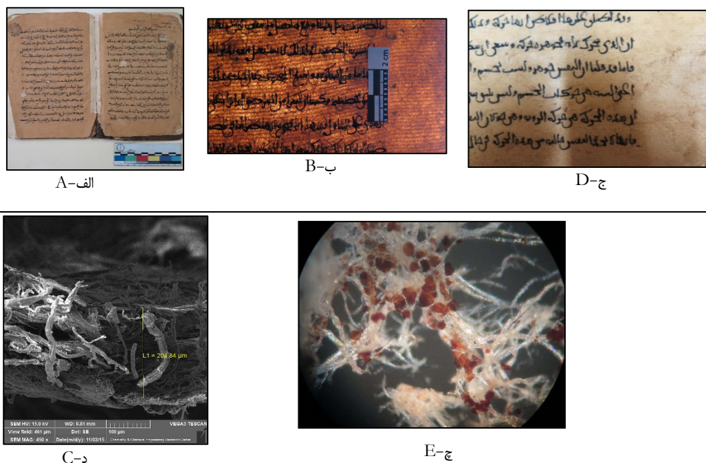
شکل ۲. کاغذ ترمه ۵۹۲۲- T: الف) کاغذ به رنگ قهوه‌ای؛ ب) عدم پراکندگی یکنواخت خمیر کاغذ، انحراف خطوط موازی قالب از راستای مستقیم، فاصله خطوط ۱-۲/۱ mm به تعداد ۷ عدد در ۱ cm؛ ج) و د) لکه‌های قرمز رنگ، کاغذ به ضخامت ۰/۲۰ mm
