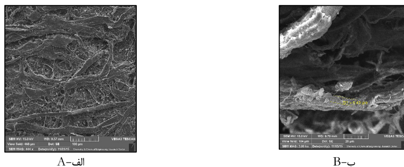
شکل ۱۰. تصاویر SEM از الیاف کاغذ T-۵۹۲۲: الف) پوشش سطحی آهار نشاسته برنج و مهره‌کشی در بزرگنمایی ۴۴۴X؛ ب) اندازه ضخامت پوشش آهار در مقطع عرضی و اندازه گرانول‌ها در بزرگنمایی ۲ KX
