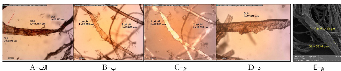
شکل ۵. الیاف پوستی و سلول‌های همراه شاهدانه در خمیر کاغذ D-۳۴۵ در بزرگنمایی ۱۰۰ X و ۲۰۰ X: (الف) و (ب) فیبرهای پوستی؛
