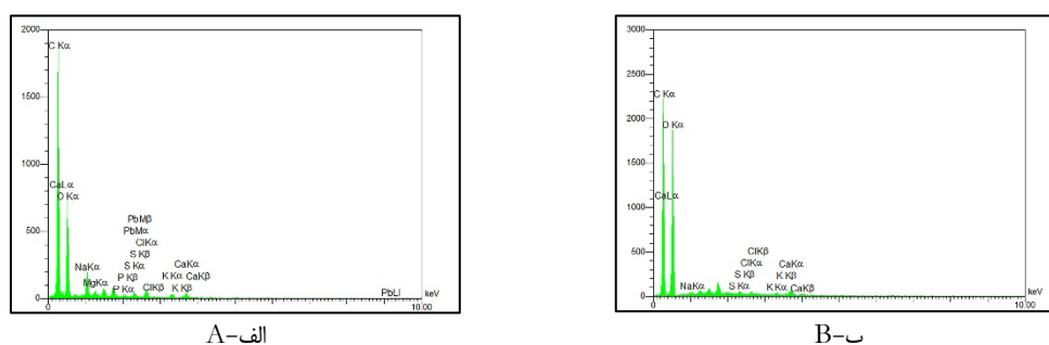
شکل ۱۱. نمودار آنالیز عنصری EDX: الف) کاغذ ۳۴۵-D؛ ب) کاغذ ۵۹۲۲-T Figure 11. Diagram of EDX elemental analysis: A) D-345 paper and B) T-5922 paper
