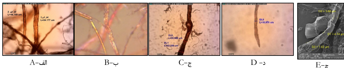
شکل ۶. الیاف کتان و شاهدانه در خمیر کاغذ ۵۹۲۲ T- در بزرگنمایی \times 100 : الف) الیاف با ضخامت‌های مختلف و حفره لومن متفاوت؛ ب) بندها در لیف باریک و خطوط متقاطع فراوان در لیف پهن در نور پلاریزان؛ ج) لیف با راستای مستقیم؛ د) انتهای لیف؛ ج) تصویر SEM الیاف با بزرگنمایی \times 5000
