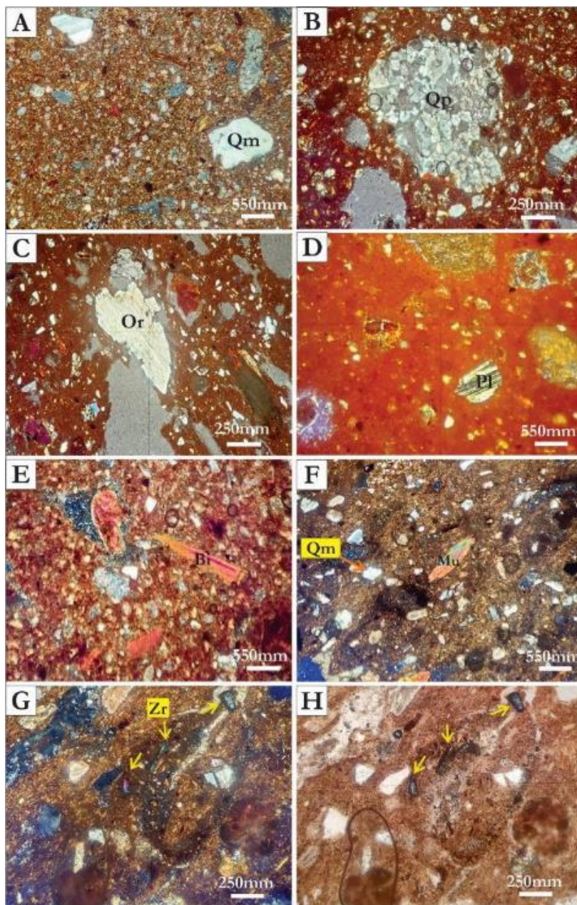
شکل ۴: تصاویر میکروسکوپی از انواع مواد افزودنی تشکیل‌دهنده سفال‌های مورد مطالعه، (A) کوارتز، تک‌بلور و لکانیکی (Qm)، (B) کوارتز چند بلور دگرگونی، تبلور مجدد (Qp)، (C) فلدسپات ارتوکلاز (Or)، (D) فلدسپات پلاژیوکلاز (Pl)، (E) میکای بیوتیت (Bi)، (F) میکای مسکویت (Mu) و کوارتز، تک‌بلور پلوتونیک (Qm)، (G) کانی سنگین شفاف زیرکان (Zr) (تصاویر A تا G در نور پلاریزه متقاطع عکس‌برداری شده است) و (H) همان تصویر G در نور پلاریزه موازی، برجستگی کانی زیرکان نسبت به اجزاء دیگر کاملاً مشخص است (در بزرگنمایی‌های ۵X و ۱۰X).
