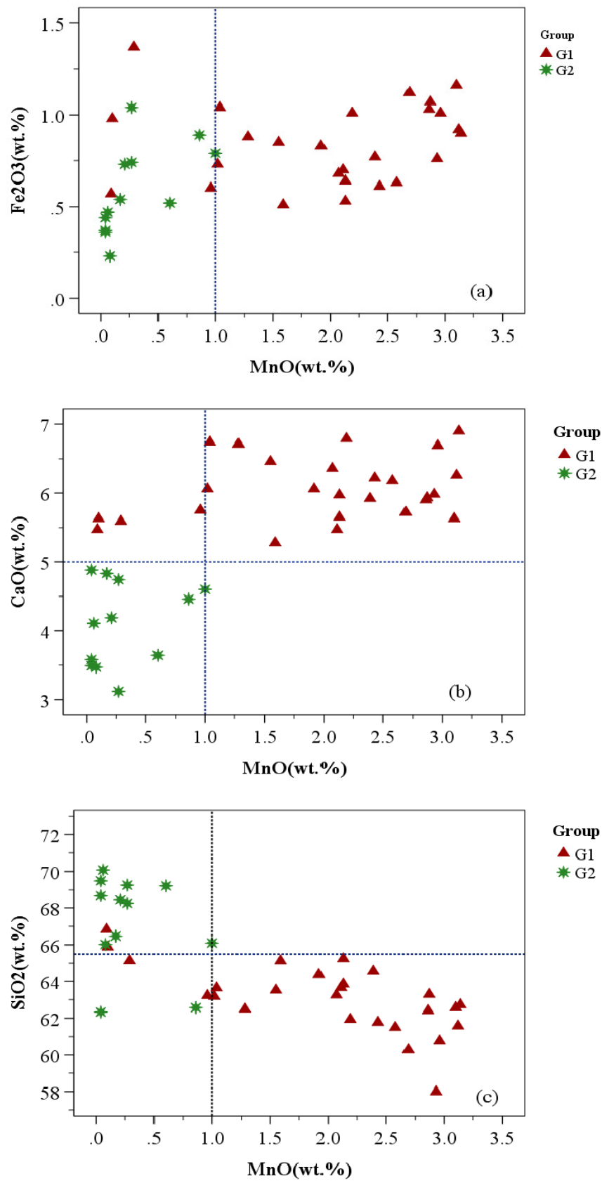
تغییرات اکسید منگنز برحسب اکسید آهن (a)، تغییرات اکسید منگنز برحسب اکسید کلسیم (b)، تغییرات اکسید منگنز برحسب اکسید سیلیسیم (c) در نمونه‌های آنالیز شده از سیمره
