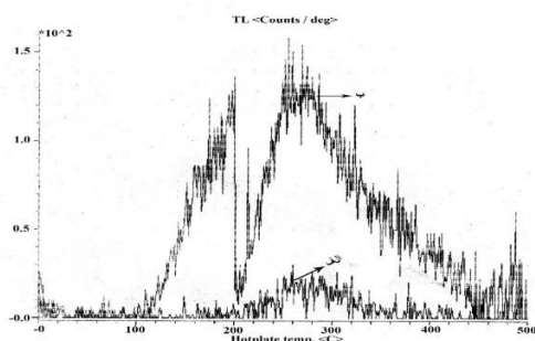
شکل ۱۲. نتایج ترمولومینسانس آجر سقافار وسطی کالا. الف- نمودار ترمولومینسانس طبیعی نمونه ب- نمودار ترمولومینسانس نمونه پس از پرتودهی با چشمه‌ی بتا.
