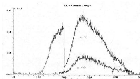
شکل ۱۱. نتایج ترمولومینسانس آجر سقانفار سید ابوصالح. الف- نمودار ترمولومینسانس طبیعی نمونه ب- نمودار ترمولومینسانس نمونه پس از پرتودهی با چشمه‌ی بتا.
