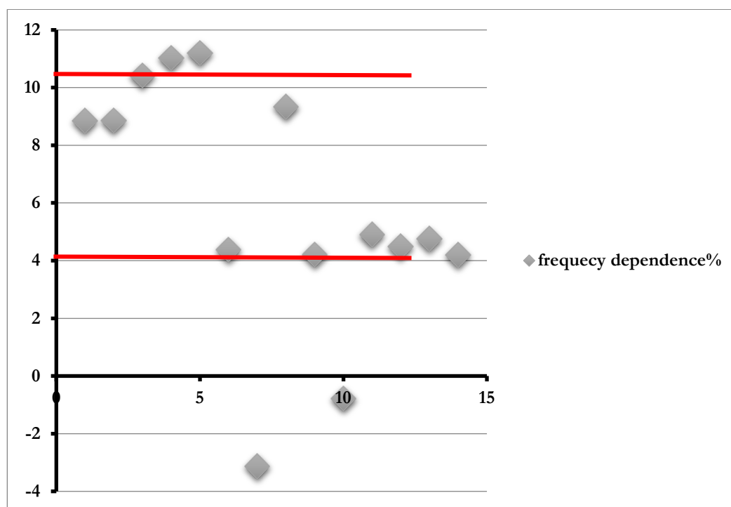
شکل ۹. نمودار پراکندگی کانی‌های فرو مغناطیسی بر اساس اندازه دانه‌های مغناطیسی Figure 9. Scatter plot of ferromagnetic minerals based on magnetic grain size.
