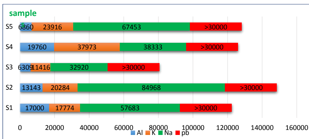
شکل ۷: نمودار مقایسه‌ی مقداری عناصر قلیایی، آلومینیوم و سرب در نمونه‌های لعاب مورد مطالعه Fig. 7: Comparison diagram of some alkaline elements, aluminum and lead in the studied glaze samples
