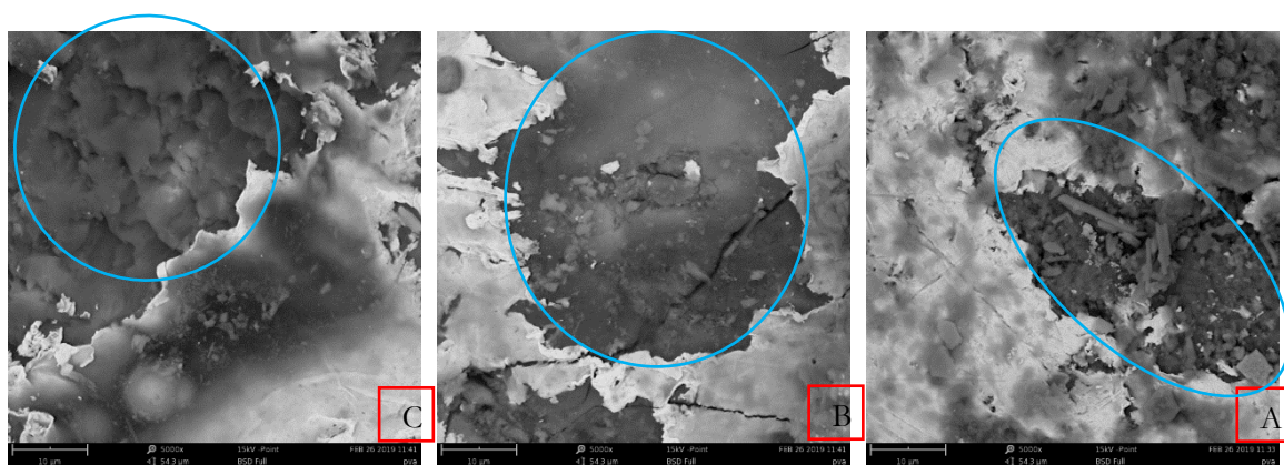
شکل ۹: ورق طلا و لایه‌های زیرین. A و B: لایه اول (دوره شاه تهماسب); C: لایه دوم (دوره شاه عباس) Fig. 9: Gold leaf and underlays. A and B: The first layer (Shah Tahmaseb's period); C: Second layer (Shah Abbas period)
