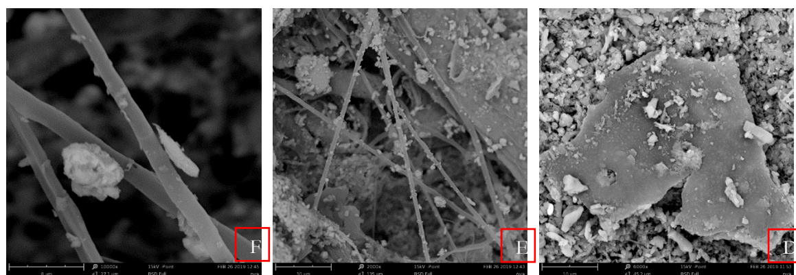
شکل ۱۰: ساختار لایه‌چینی. D: لایه اول (دوره شاه تهماسب); E و F: لایه دوم (دوره شاه عباس) Fig. 10: Pastiglia structure. D: The first layer (Shah Tahmaseb's period); E and F: second layer (Shah Abbas period)
