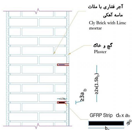
شکل ۸: نحوه قرارگیری نوارهای GFRP در دیوارهای بنایی Fig. 8: Configuration of GFRP strips in masonry walls
