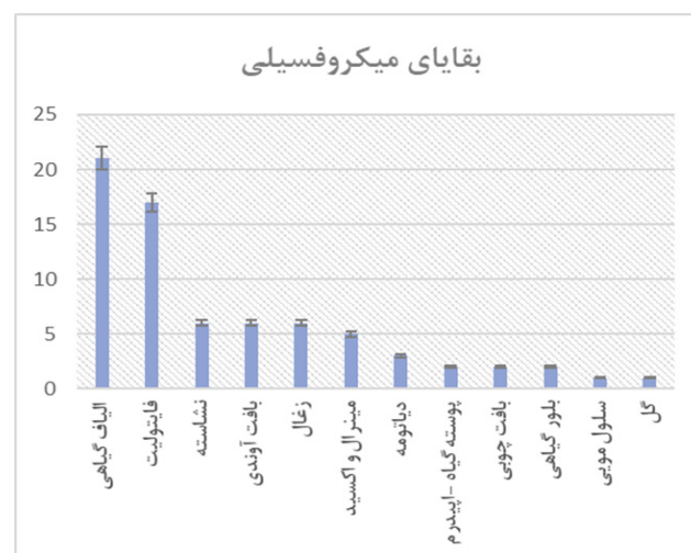
شکل ۱۲. بقایای میکروفسیلی به دست آمده از سنگ‌ساب‌های صخره‌ای باوه‌یوان. Figure 12. Microfossil remains obtained from the rock fragments of Baoheyuan.
