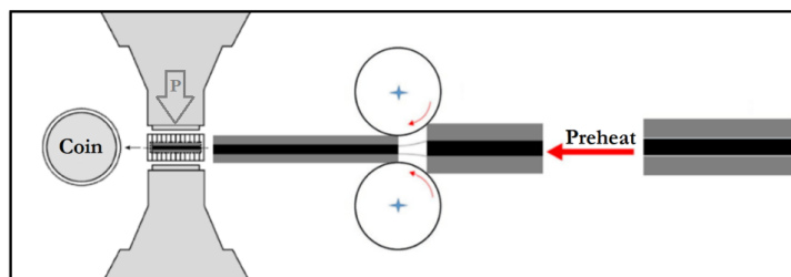
شکل ۱۱. الف) تصویر شماتیک از فرایند نورد اتصالی به همراه فرایند سکه‌زنی Figure 11. Schematic picture of roll bonding process along with minting process
