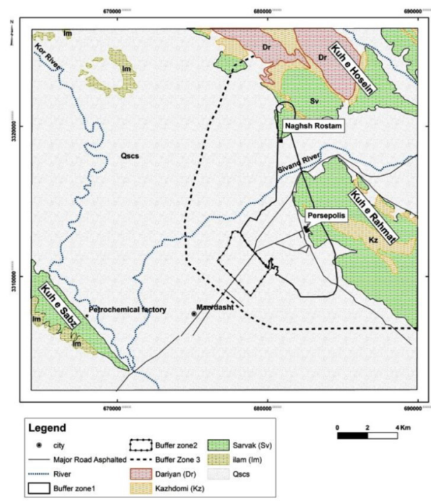
شکل ۲. نقشه زمین‌شناسی منطقه مورد مطالعه به همراه سازندهای مختلف و موقعیت نقش‌رستم و مجتمع پتروشیمی (رئیزی اردکانی، ۱۳۸۹)
