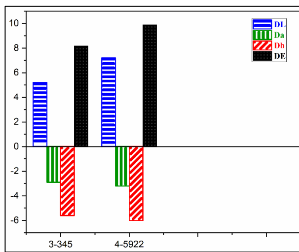
شکل ۴. نمودار تغییرات رنگی بین کاغذهای آهاردار و بدون آهار D-۳۴۵ و T-۵۹۲۲ Figure 4. Diagram of color changes between sizing and non-sizing papers D-345 and T-5922
