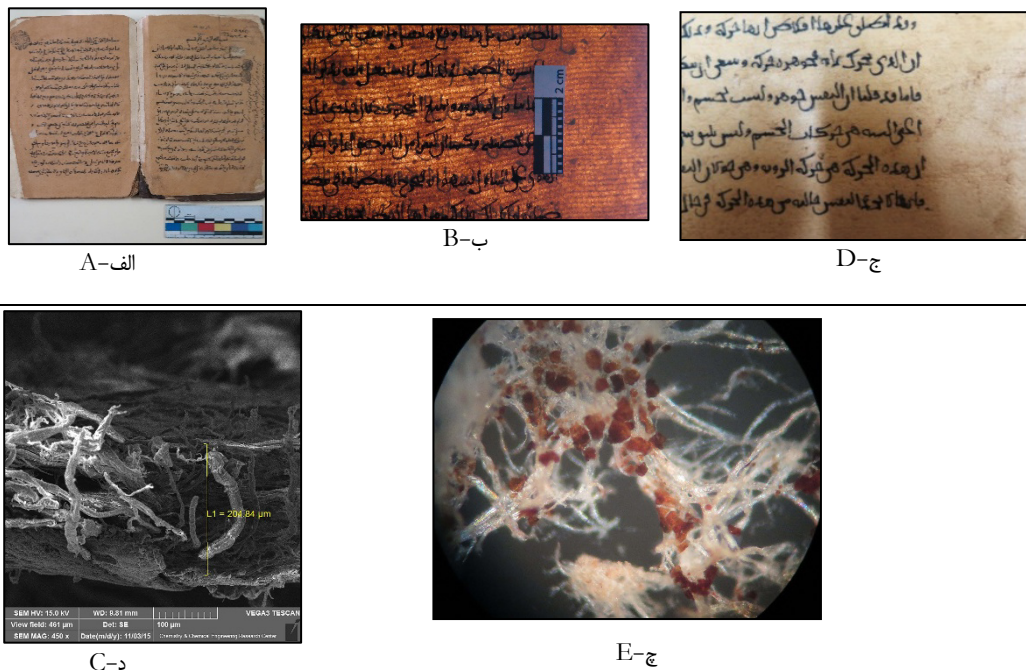
شکل ۲. کاغذ ترمه ۵۹۲۲- T: الف) کاغذ به رنگ قهوه‌ای؛ ب) عدم پراکندگی یکنواخت خمیر کاغذ، انحراف خطوط موازی قالب از راستای مستقیم، فاصله خطوط ۱-۲/۱ mm به تعداد ۷ عدد در ۱cm؛ ج) و د) لکه‌های قرمز رنگ، کاغذ به ضخامت ۰/۲۰ mm
