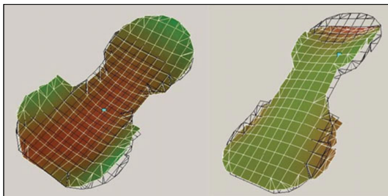
شکل ۸. تلفیق حالت‌های ارتعاش صفحات ویلن به‌دست‌آمده با اسکن ویبرومتری لیزری و آنالیز مدها، عکس از کتاب ویوچیتا بوچورا، به نقل از مدرسه عکاسی مهندسی و فناوری اطلاعات، دانشگاه نیو ساوت ولز، کانبرا، استرالیا (Bucur, 2016, p. 141)
