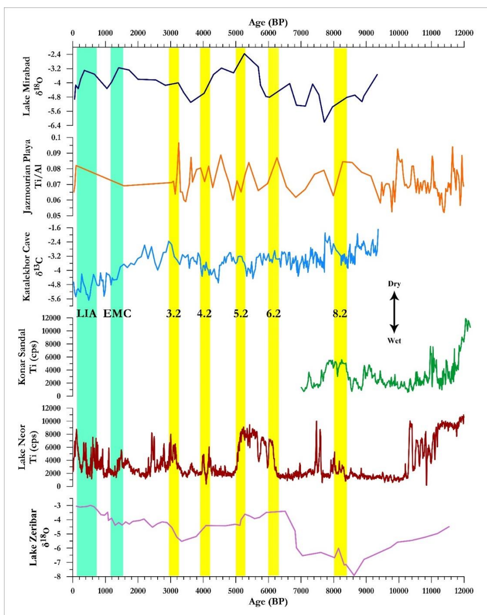
شکل ۲: نوسانات اقلیمی در عصر هولوسن. نوارهای زرد نشان‌دهنده رویدادهای اقلیمی خشک و نوارهای آبی نشان‌دهنده دوره‌های سرمایش اوایل قرون وسطی (EMC) و عصر یخبندان کوچک (LIA) هستند. دریاچه زیربار (Stevens, Wright Jr, & Ito, 2001)، دریاچه نئور (Sharifi et al., 2015)، کنار صندل جیرفت (Safaierad et al. 2020)، غار کتله خور (Andrews et al., 2020)، جازموریان پلایات (Vaezi et al., 2019)، دریاچه میرآباد (Stevens, Ito, Schwalb, & Wright, 2006)، دریاچه ارومیه (Sharifi et al., 2023).
