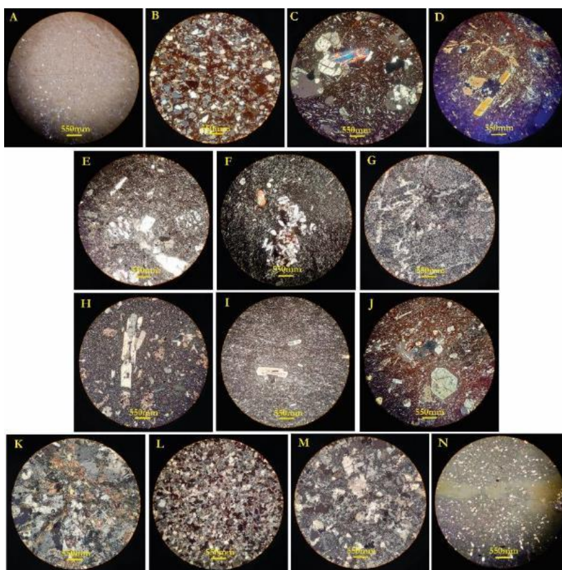
شکل ۹: تصاویر میکروسکوپی (نور پلاریزه متقاطع و بزرگمایی ۵X) سنگ‌ریزه‌های پراکنده در سطح و اطراف محوطه گبری مود، (A) مادستون، (B) ماسه‌سنگ آهکی، (C) پیروکسن آندزیت، (D) آندزیت بازالتی، (E) داسیت، (F) آندزیت بازالتی، (G) سرپانتینیت، (H) آندزیت، (I) داسیت، (J) پیروکسن آندزیت، (K) بازالت، (L) ماسه‌سنگ آهکی، (M) بازالت، (N) مادستون ماسه‌ای
