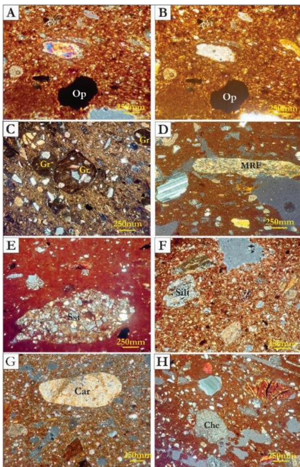
شکل ۵: تصاویر میکروسکوپی از انواع مواد افزودنی شناسایی شده (بزرگنمایی ۱۰×)، (A) کانی سنگین تیره (احتمالاً مگنتیت) (Op) نور پلاریزه متقاطع، (B) همان تصویر در نور پلاریزه موازی، کانی سنگین اپاک در هر دو نور تیره هستند، (C) گراگ یا خرده سفال (Gr)، (D) خرده سنگ دگرگونی اسلیتی (MRF)، (E) خرده سنگ رسوبی ماسه سنگی (Sst)، (F) خرده سنگ رسوبی سیلتستونی (Silt)، (G) خرده سنگ رسوبی کربناته (Car) و (H) خرده سنگ رسوب چرتی (Che)، تصاویر C تا H در نور پلاریزه متقاطع عکس‌برداری شده است.
