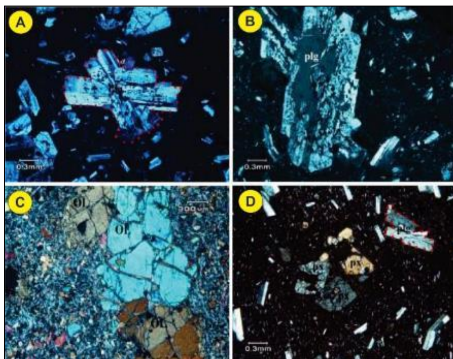
شکل ۱۱: تصویر میکروسکوپی (نور پلاریزه متقاطع و بزرگنمایی ۱۰X) از ترکیب برخی سنگ‌های آتشفشانی فراوان در اطراف محدوده مورد مطالعه (Habibi et al., 2022, p. 263-264) (A) آندزیت بازالتی، (B) آندزیت، (C) بازالت و (D) داسیت
