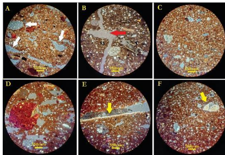
شکل ۷: تصاویر میکروسکوپ پلاریزان (نور پلاریزه متقاطع و بزرگنمایی ۵X) از حفره‌های موجود در سفال‌های مورد مطالعه، (A) روزن‌های با اشکال نامنظم، (B) کانال‌های کشیده با دیواره‌های موازی، (C) منافذ در اندازه متوسط، (D) فضاهای خالی در اندازه درشت، (E) رشد بلورهای کلسیت در حاشیه دیواره حفره‌های کانالی، (F) پرشدگی برخی روزن‌ها توسط بلورهای درشت کلسیت
