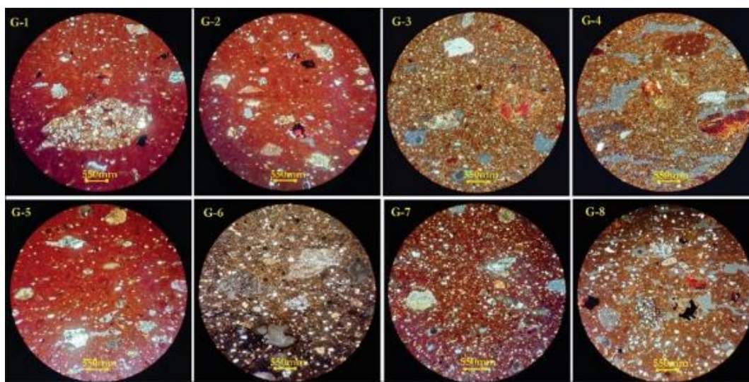
شکل ۳: تصاویر میکروسکوپی سفال‌های محوطه گبری مود (نور پلاریزه متقاطع و بزرگمایی ۵X) که اجزاء تشکیل‌دهنده خمیره‌ی آنها، به‌ویژه ماتریکس رسی در رنگ‌های مختلف قابل مشاهده است.
