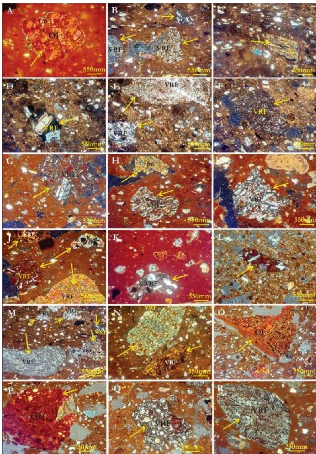
شکل ۶: تصاویر میکروسکوپی (نور پلاریزه متقاطع) از انواع خرده سنگ‌های آذرین (حد واسط و ولکانیکی) (VRF) و قطعات سنگی سرپانتینیت (Se) و کانی الیوین (Ol) در بزرگنمایی‌های ۵X و ۱۰X.
