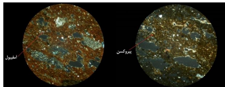
شکل ۱۱: تصویر میکروسکوپی از نمونه 16-114 و 107-122، نور XPL، کانی آمفیبول و پیروکسن
