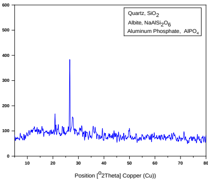
شکل ۴: طیف XRD نمونه C116-37 و نمونه L114-2
