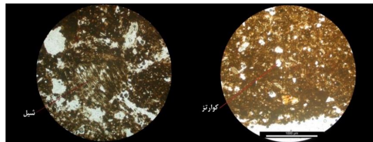
شکل ۱۲: تصویر میکروسکوپی از نمونه 2-114، نور PPL، شیل و کوارتز در مرکز تصویر
