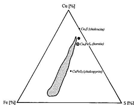
شکل ۳: فاز سه‌تایی Cu-Fe-S، نشان دهنده منطقه تجزیه مات و رسوب مس برای دماهای بین 185^\circ\text{C} و 548^\circ\text{C} . علائم ● نشان دهنده مات و ■ نشان دهنده شکاف امتزاج‌پذیری: ناحیه تجزیه مات و رسوب مس [49].
