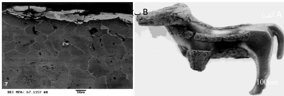
شکل ۹: الف) تصویر SEM از گاو هورز تپه که وجود فاز \gamma به صورت گسترده در سطح نشان‌دهنده پوشش سماتاسیون در سطح این اثر است. ب) گاو به دست آمده از هورز تپه.
