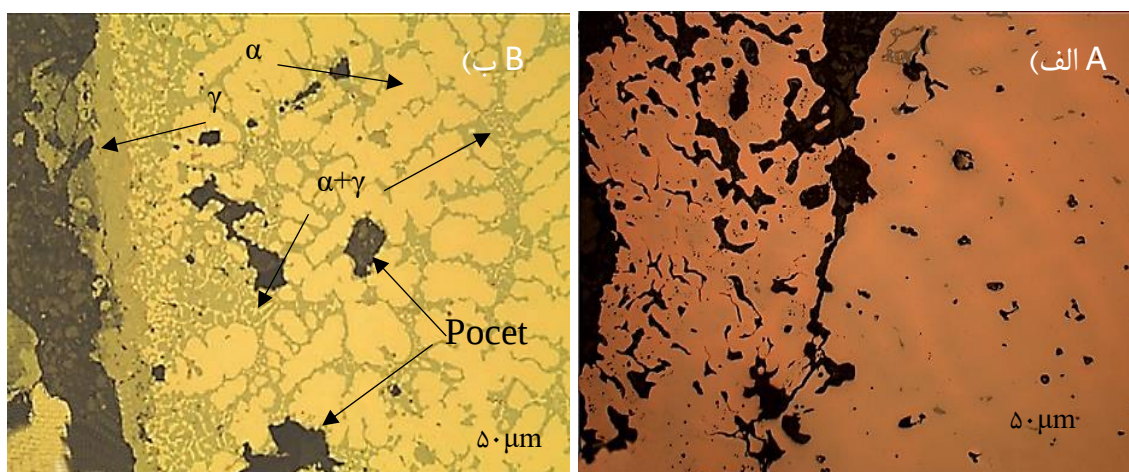
شکل ۷: الف) ساختار برنز آرسنیک بعد از نیم ساعت در اثر بخار آرسنیک، شکاف و یا پاکت‌هایی ایجاد شده است [104].
