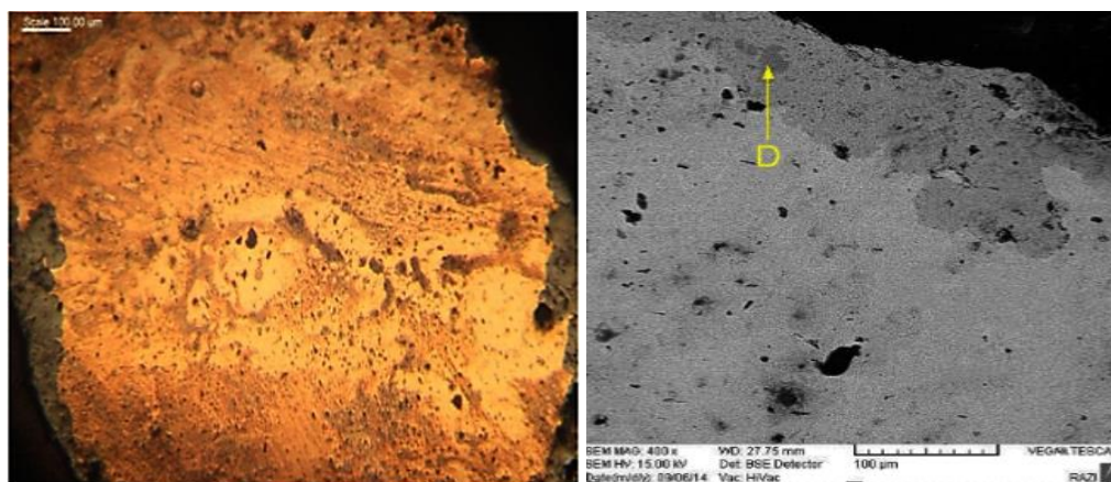
شکل ۱۰: خوردگی تعمدی برای پوشش نقره‌ای رنگ در اولین نمونه گوشواره به دست آمده از جعفرآباد گرگان (J-A-2010-35) [116] Fig. 10: Intentional corrosion for silver coating in the first earring sample obtained from Jafarabad, Gorgan (J-A-2010-35) [116]
