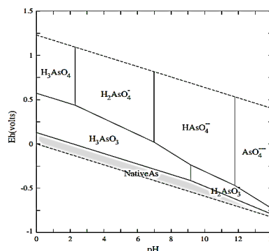
شکل ۱: دیاگرام Eh-pH برای سیستم As-O-H در 25^\circ\text{C} و فشار 1 Bar. \Sigma\text{As} تنظیم شده است.
