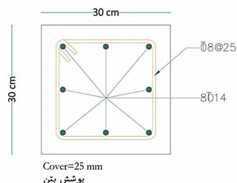
شکل ۷: کلاف بتنی افقی مورد استفاده در بالای دیوارهای بنایی Fig. 7: Concrete tie beam at the top of the masonry walls
