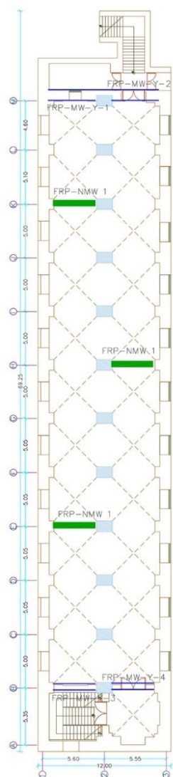
پلان طرح مقاومسازی زیرزمین
