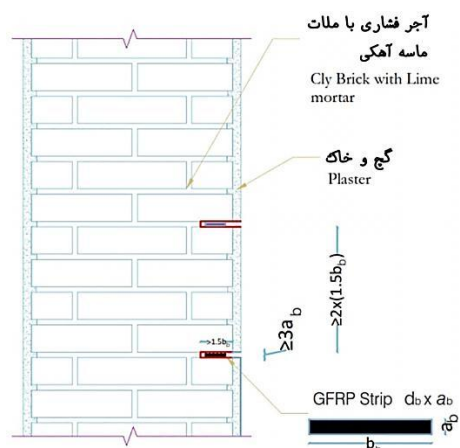
شکل ۸: نحوه قرارگیری نوارهای GFRP در دیوارهای بنایی Fig. 8: Configuration of GFRP strips in masonry walls
