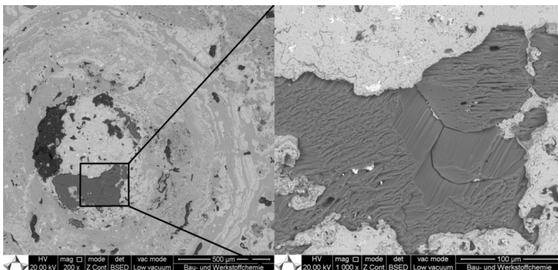
شکل ۷: نوک نمونه به همراه تجمع آهک یا کلسیت در زیر لایه خوردگی. دانه‌های با نور منعکس به بالا، ذرات سربی هستند.
