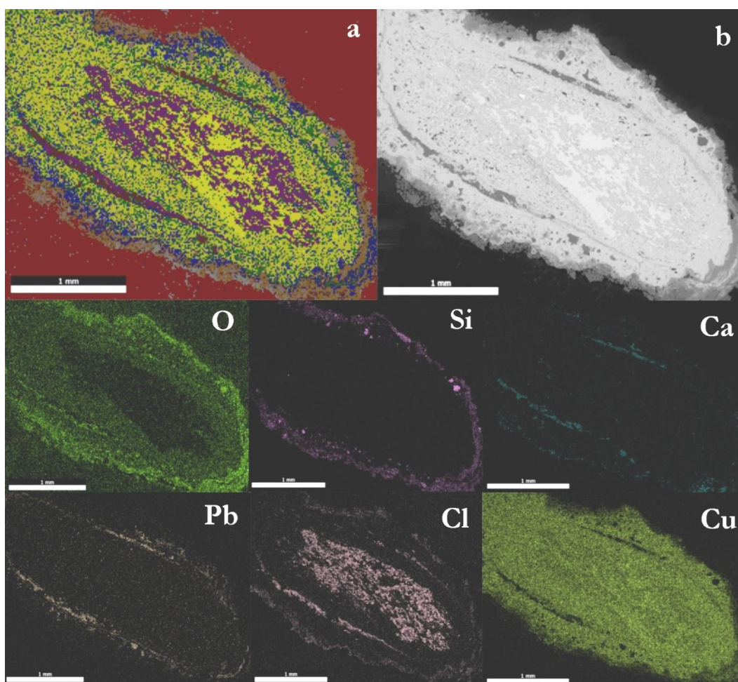
شکل ۸: (a) تصویر اسکن عنصری انتهای قلم فلزی با استفاده از میکروسکوپ الکترونی و (b) تصویر الکترونی خالص سطح به همراه اسکن ردیابی وجود عناصر O, Si, Ca, Pb, Cl, Cu Fig. 8: A) Scanning electron image of the bottom of pin. B) Scanning electron image of the surface with the trace of such elements as Cu, Cl, Pb, Ca, Si, O.
